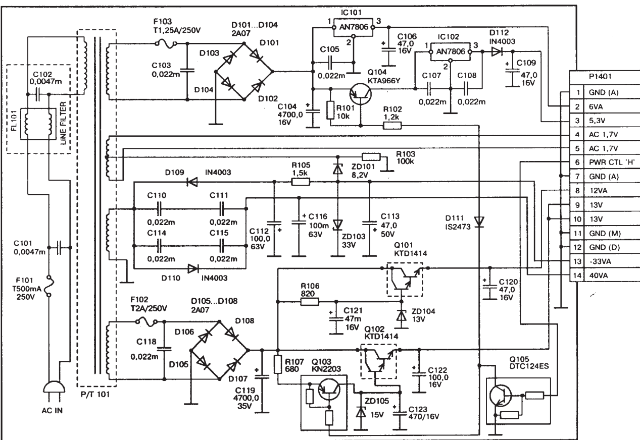
Принципиальная схема источника питания видеомэагнитофона SV-T21 фирмы SUPRA.
